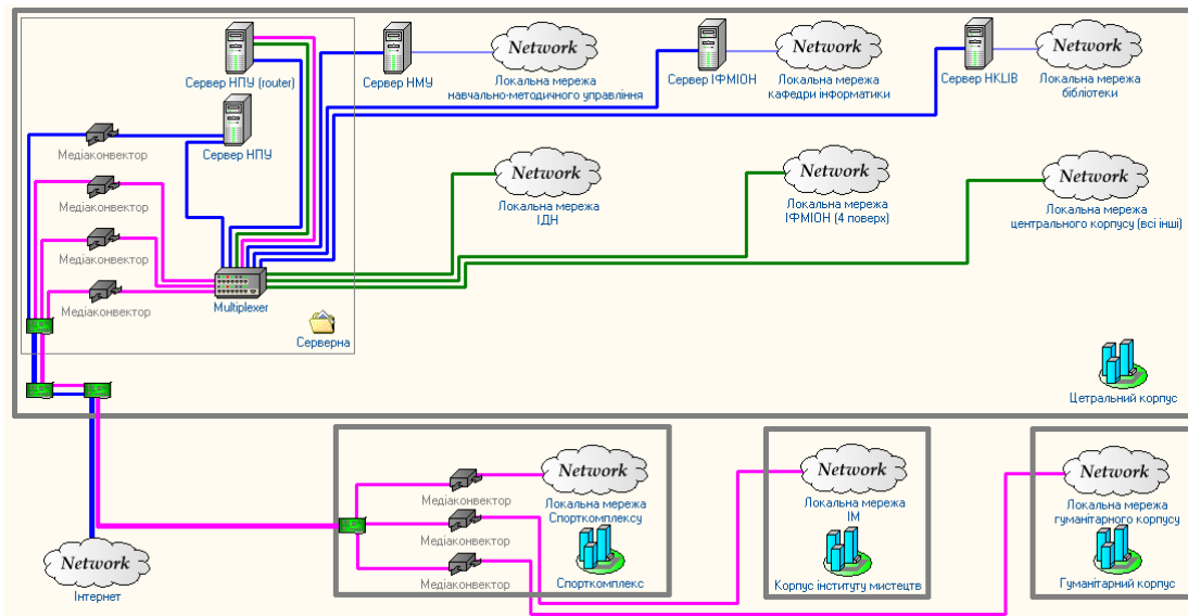
Рис. 6.3.2. Мережа Інтранет університету
